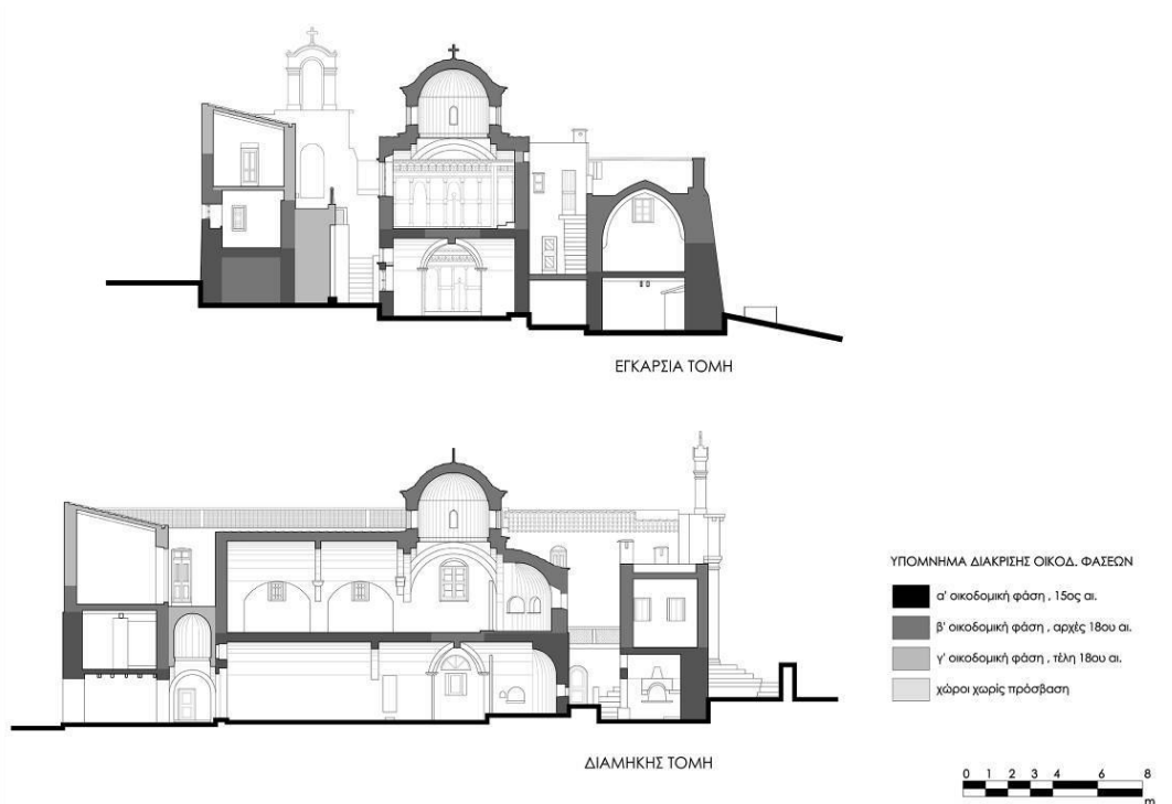
Εικ. 6: Διάγραμμα Εγκάρσιας και Διαμήκουσ Τομής του συγκροτήματος.
